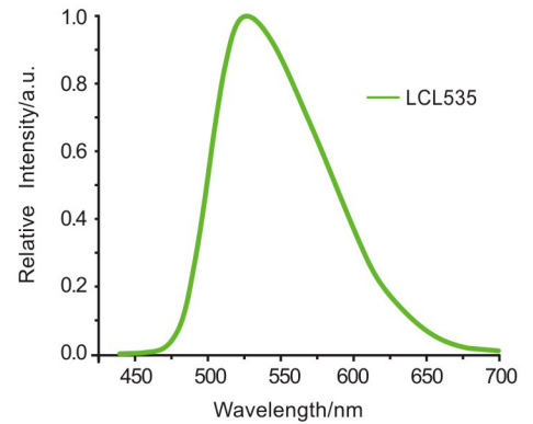
发射光谱 EM Spectrum
